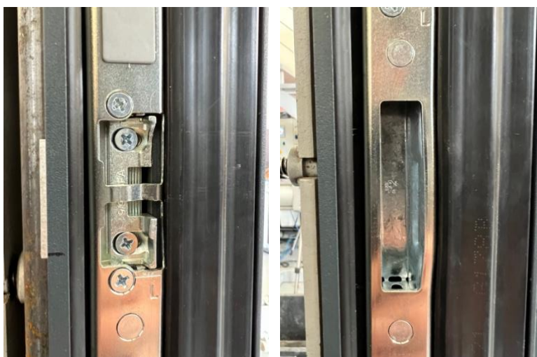
Obiekt badań Nr 1. Badanie odporności na obciążenie statyczne. Widoczne uszkodzenia po badaniu.
