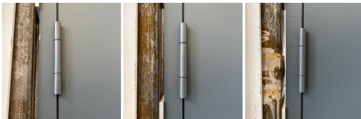
Fot. 21, 22, 23 Zawiasy od strony zewnętrznej widok od góry skrzydła do dołu.
